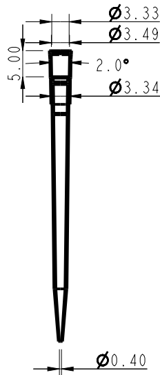
截面 A-A
